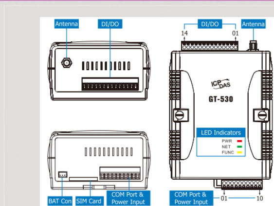
腳位規劃圖
