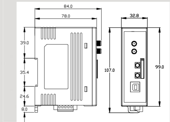
尺寸圖
