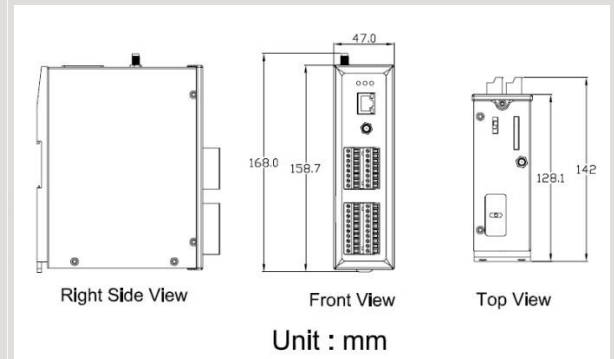
Dimensions
